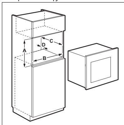
Αποστάσεις εγκατάστασης
